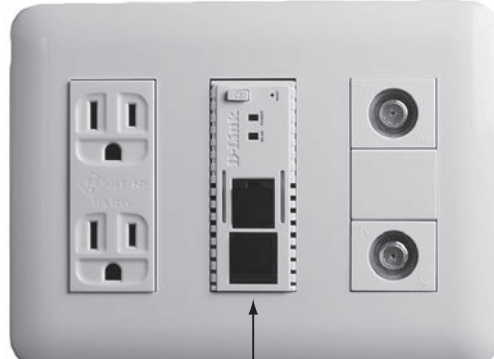
3連スイッチボックスへの取付例 ※電源/アンテナ端子/枠などはお客様準備
